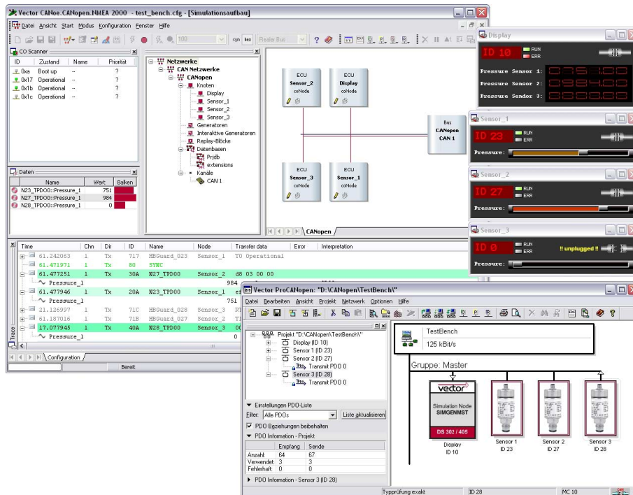
[Bild 2: Eine wesentliche Erleichterung bei der Busanalyse stellt die farbige Unterscheidung verschiedener CANopen-Dienste im Trace-Fenster dar.]
