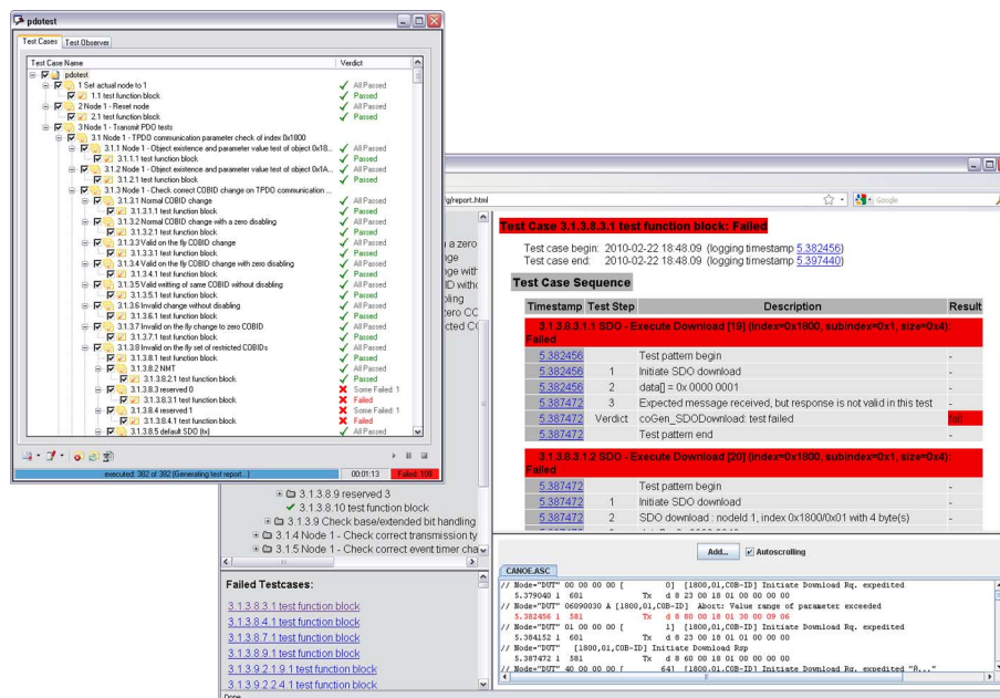
[Bild 1: Mit CANoe.CANopen spezifiziert der Anwender protokollspezifische Tests einfach und generiert diese auf Knopfdruck. Beim Ausführen eines Testmoduls wird ein umfangreiches Testprotokoll erzeugt.]
